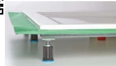
superflache Duschwanne mit Montagerahmen inkl. Randverstärkung + Dichtvlies (Höhe Wannenrand 1,5 cm)
